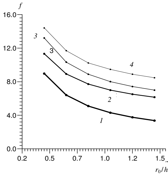
Рис. 3. Зависимость резонансной частоты f (ГГц) от формы ЦДР для однородного (1, 2) диэлектрика с \varepsilon = 50 и неоднородного вдоль оси z диэлектрика (3, 4) для h = 5 мм: 1 – мода H_{01\delta} ; 2, 3, 4 – мода H_{011}
