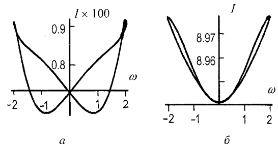
Рис. 2. Зависимость интенсивности пучка I от частоты лазера \omega при \Omega = 0.5 , \omega_1 = 2 : a – в случае слабого поля, E_0 = 0.1 ; b – в случае сильного поля, E_0 = 3
