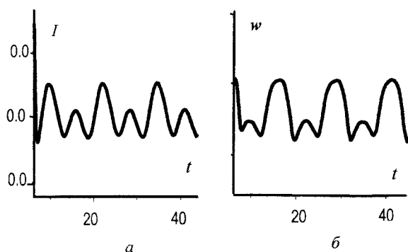
Рис.3. Интенсивность на оси пучка I (а) и размер пятна w (б) в условиях значительного насыщения, E_0 = 3 , частота модуляции \Omega = 0.5 , амплитуда модуляции \omega_1 = 1
