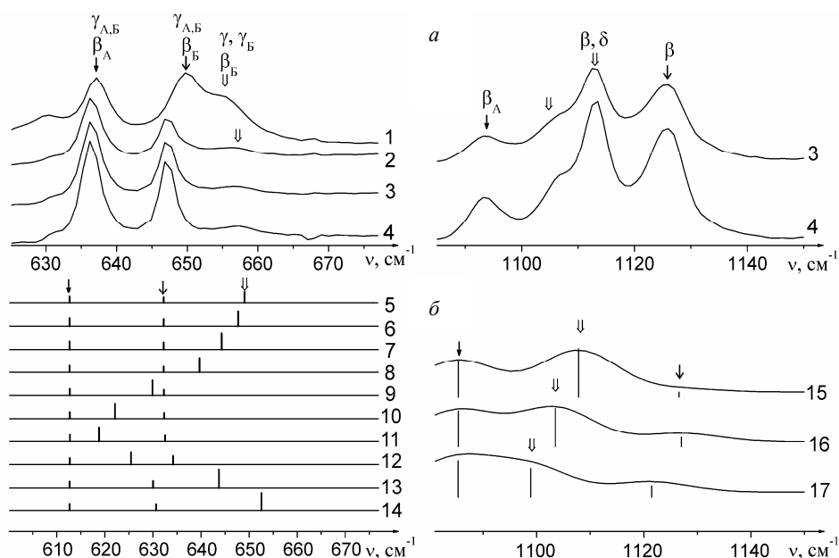
Рис. 4. ИК спектры 4ЦБ: измеренные при 55° (1), 50° (2), 48° (3) и 28° С (4) и рассчитанные для конформеров с углами \phi_3 , равными 0 (5), 10° (6), 20° (7), 30° (8), 50° (9), 70° (10), 90° (11), 120° (12), 150° (13), 180° (14) и углами \phi_4 , равными 0 (15), -41° (16), -98° (17)
