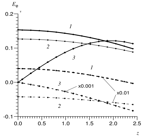
Рис. 5. Зависимость \text{Re}(E_\phi) (сплошные кривые) и \text{Im}(E_\phi) (штриховые кривые) от координаты z (мм) для ЦДР \varepsilon = 100 , r_0 = h = 5 мм: 1, 2 – мода H_{01\delta} при \rho = 3, 4 и \rho = 1.66 мм; 2 – мода H_{011} при \rho = 4.46 мм
