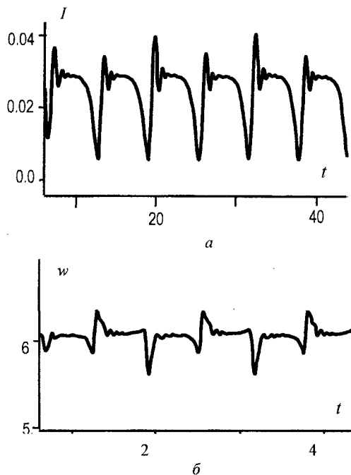
Рис. 5. Интенсивность на оси пучка I (а) и размер пятна w (б) в условиях появления нестационарных когерентных эффектов: E_0 = 3 , \Omega = 0.5 , амплитуда модуляции \omega_1 = 10
