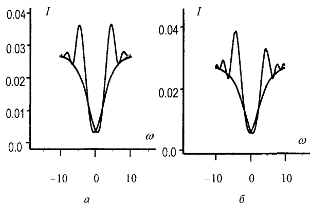
Рис. 4. Проявление нестационарных когерентных эффектов при \Omega = 0.5 , \omega_1 = 10 : а – в случае слабого поля, E_0 = 0.1 ; б – в случае сильного поля, E_0 = 3
