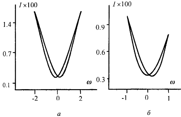
Рис. 1. Зависимость интенсивности на выходе из среды I от частоты лазера \omega : a – при отсутствии насыщения, E_0 = 0.1 , \Omega = 0.5 , \omega_1 = 2 (слабое поле); b – при умеренном насыщении, E_0 = 3 , \Omega = 0.5 , \omega_1 = 2 (среднее поле)
