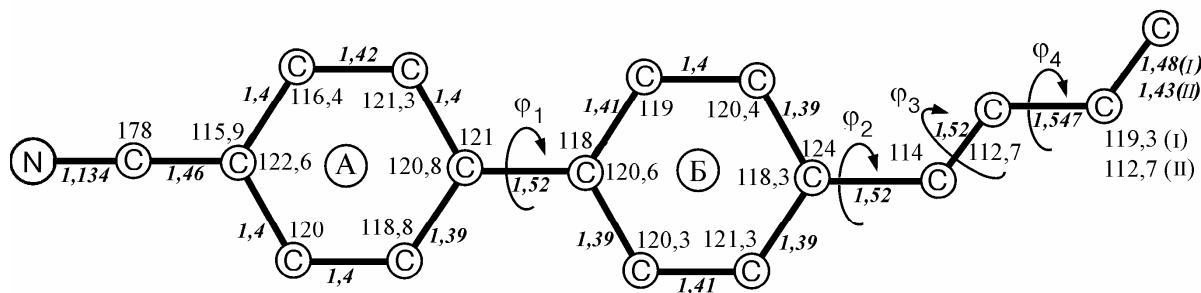
Рис. 1. Плоский конформер молекулы 4ЦБ
